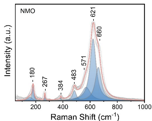
Fig.S4 Raman Spectra of NMO.
